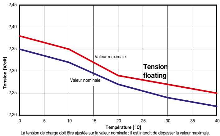
Figure 1: Marathon L/XL et Powerfit S100/S300; tension de charge en fonction de la température
